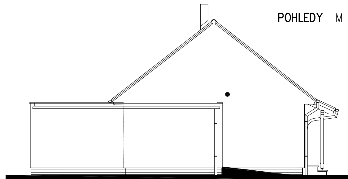
POHLED VÝCHODNÍ
