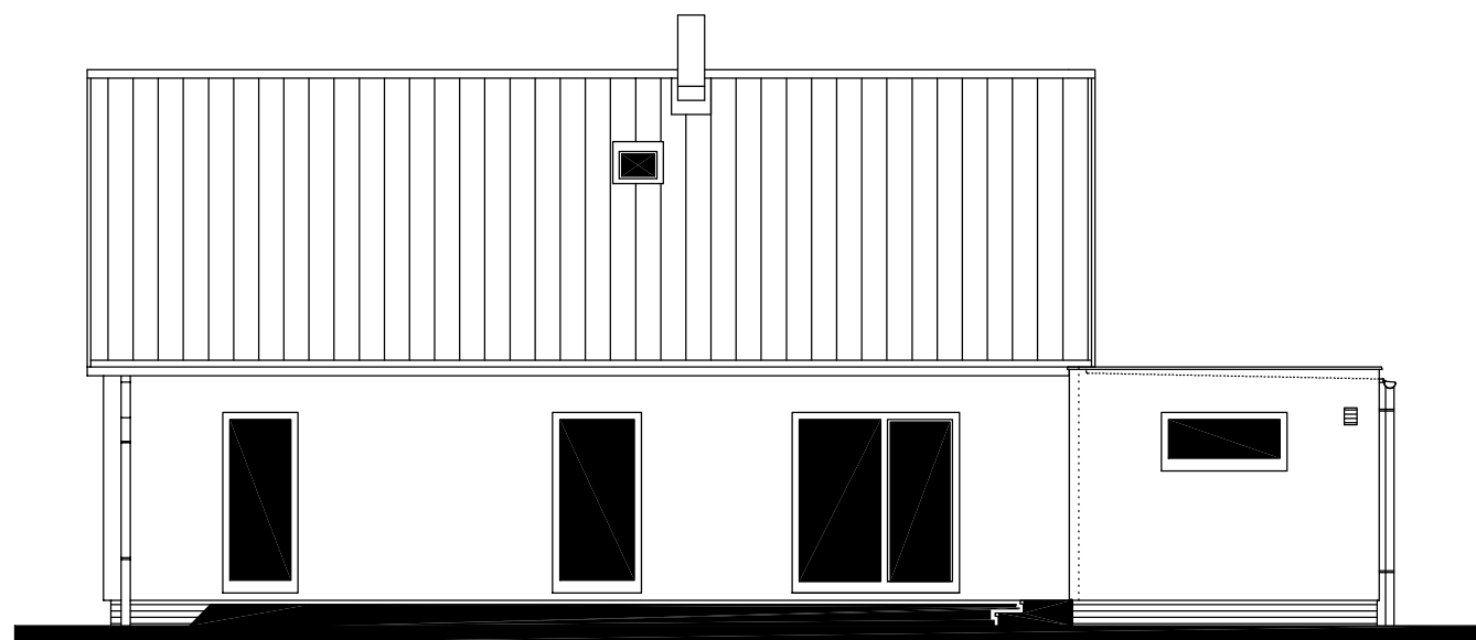
POHLED JIŽNÍ
